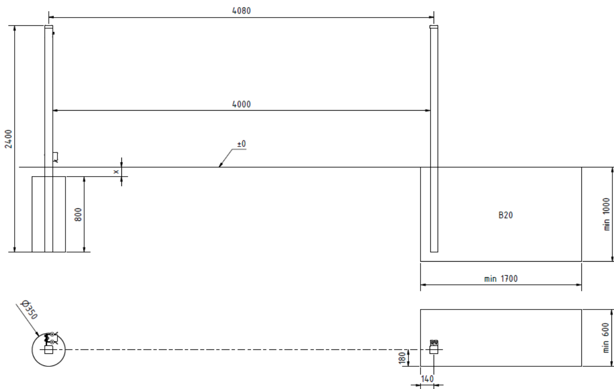
Obrázek 3 Beton + sloupky
